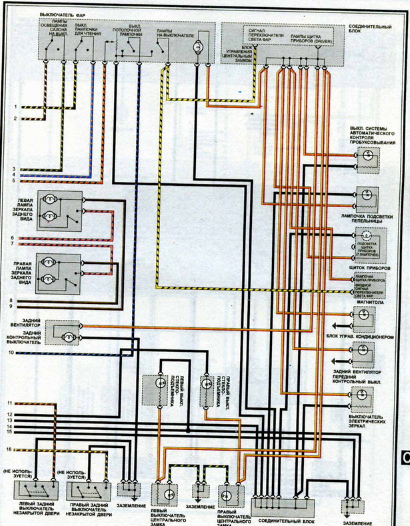
18. Типичная система освещения салона (2 из 2)
