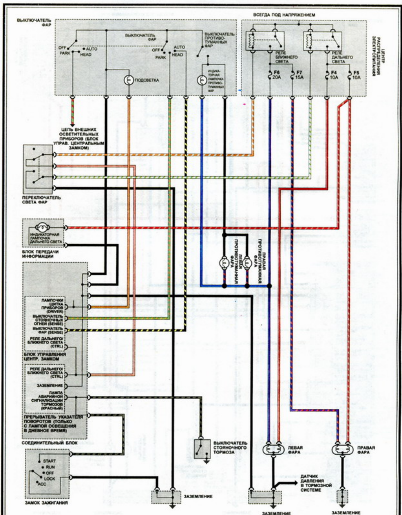
8. Типовая система фар и противотуманных фар - модели Plymouth Voyager и модели 1998 г. выпуска и более поздние Caravan
