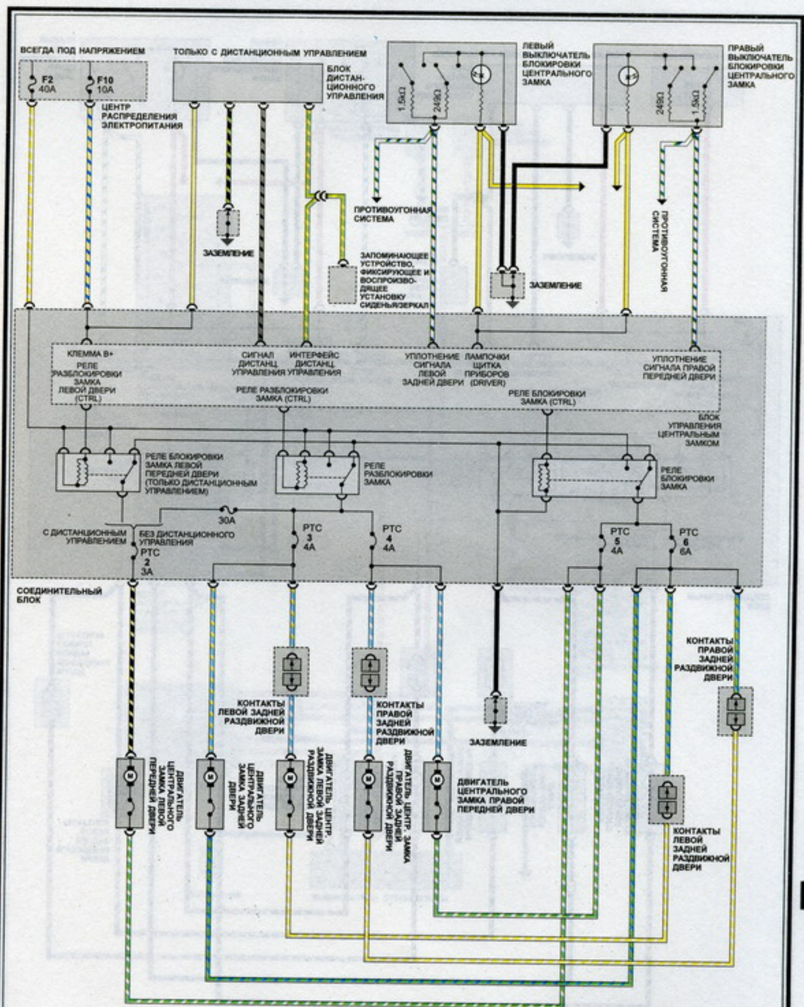
20. Центральный замок - модели 1996 и 1997 гг. выпуска
