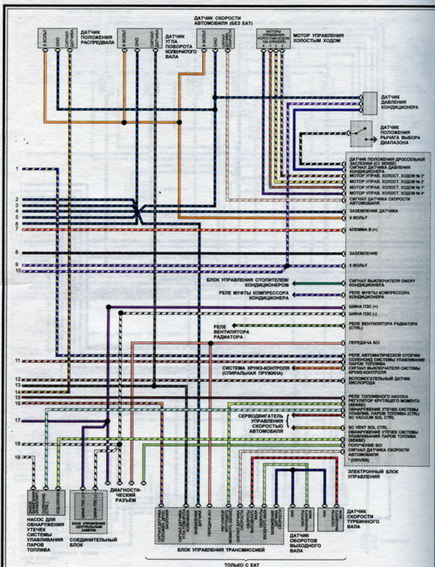
3. Типовая система управления двигателем (3 из 3)
