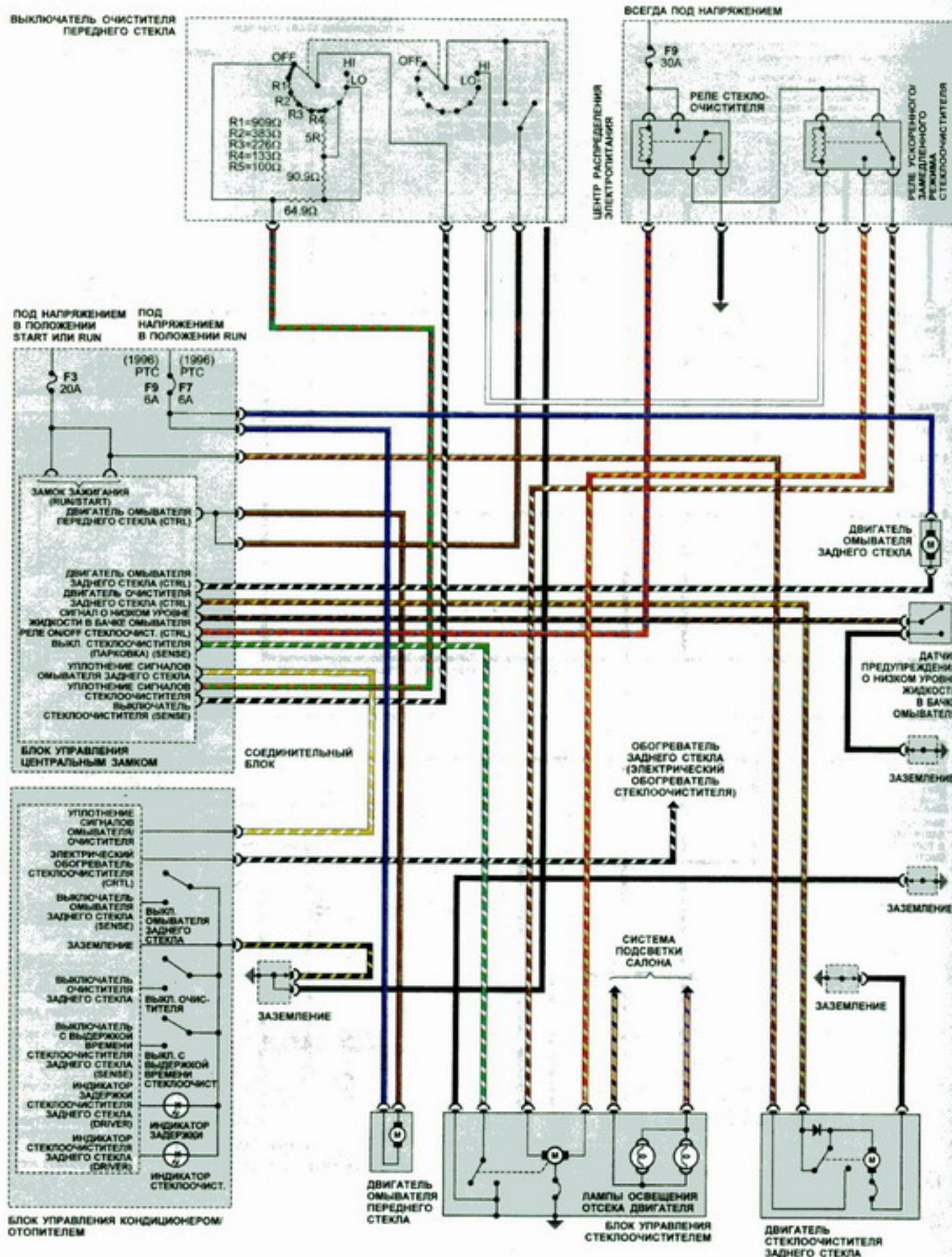
13. Стеклоочиститель ветрового стекла - модели 1996-1997 гг. выпуска
