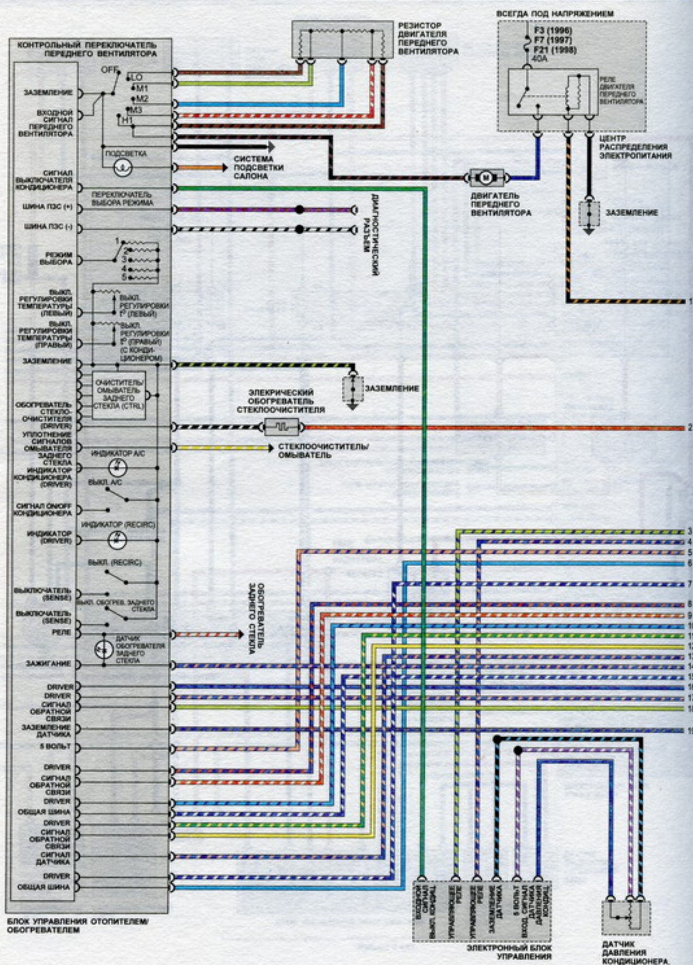
5. Кондиционер и отопитель - включая вентилятор системы охлаждения (1 из 2)
