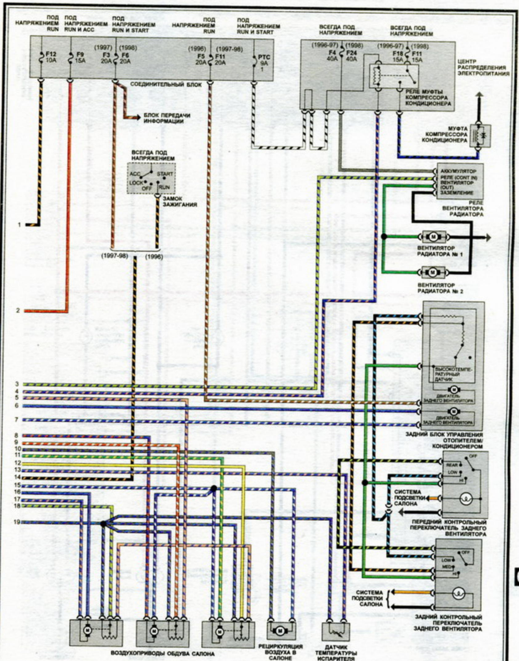
6. Кондиционер и отопитель - включая вентилятор системы охлаждения (2 из 2)
