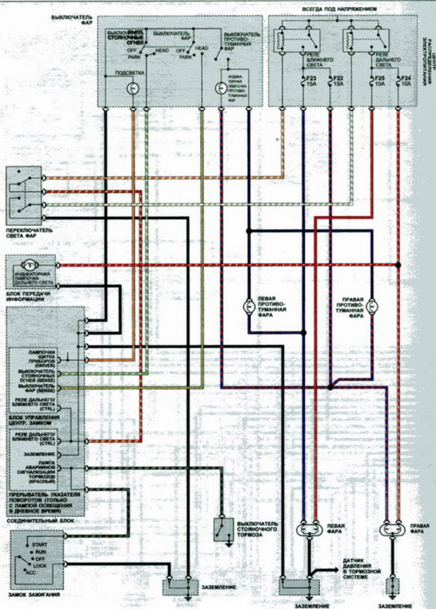
7. Типовая система фар и противотуманных фар - модели 1996 и 1997 гг. выпуска
