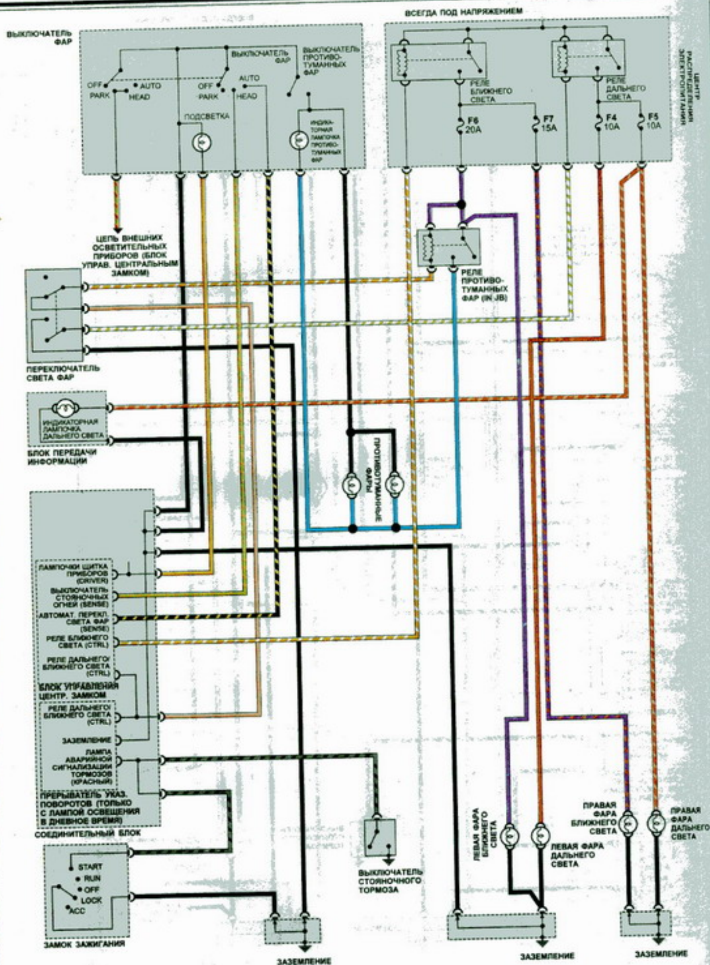
9. Типовая система фар и противотуманных фар - модели Chrysler Town & Country 1998 г. выпуска и более поздние
